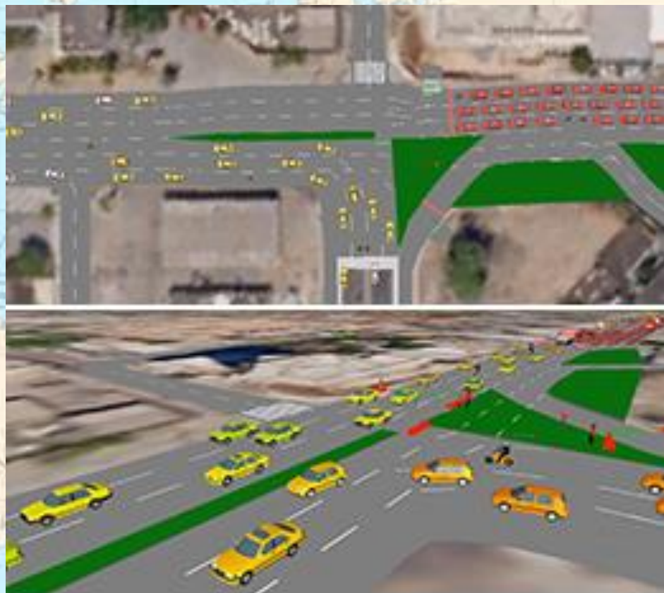
マイクロシミュレーションによる渋滞解析 (上) マイクロシミュレーションによる交差点部の解析 (下)
